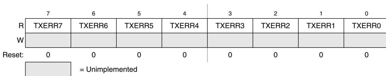
Figure 16-19. MSCAN Transmit Error Counter (CANTXERR)
